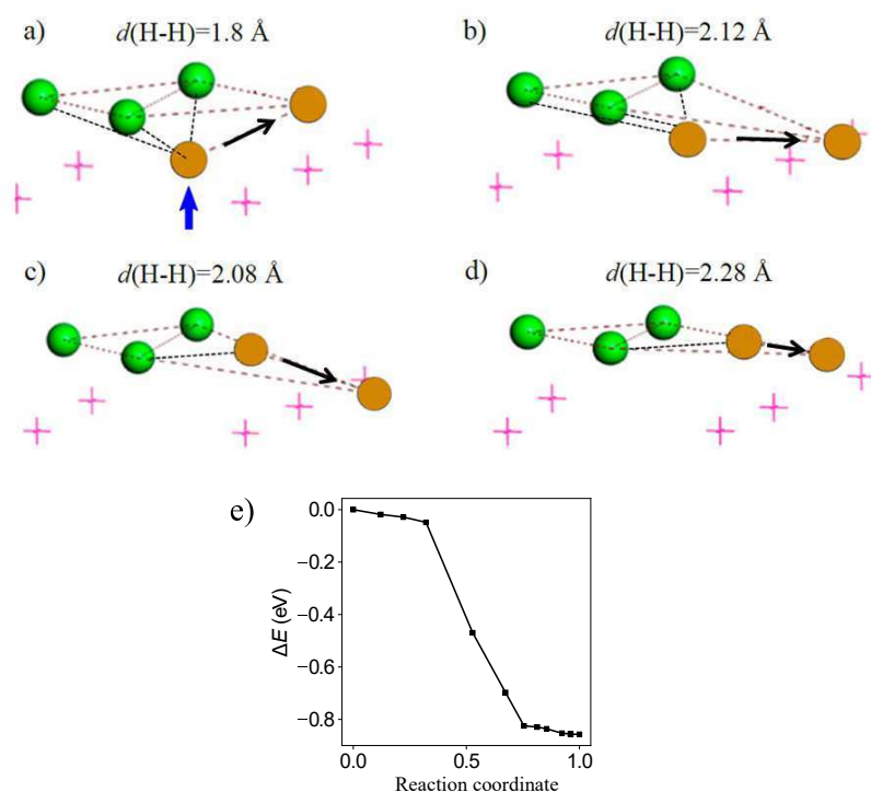
Рис. 8. a, b, c, d — Рост малого кластера за счет выхода атома Н из массива (на рис. 8 a показан синей стрелкой). Черной стрелкой показано направление выталкивания одного из атомов кластера на его периферию; e — изменение энергии системы в процессе перемещений, представленных на рис. 8 a, b, c, d (за уровень отсчета принята энергия начальной конфигурации системы, соответствующая рис. 8 a )
