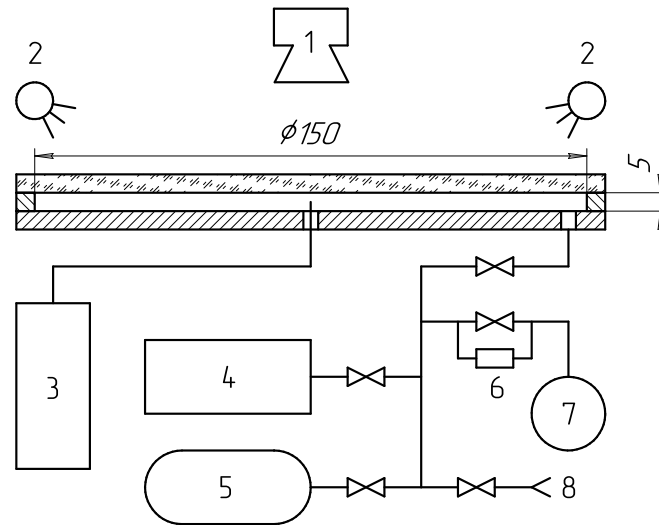
Рис. 2. Схема экспериментальной установки: 1 — видеокамера; 2 — подсветка; 3 — генератор высоковольтного разряда; 4 — вакуумный насос; 5 — баллон с водородом; 6 — дифференциальный манометр; 7 — образцовый вакуумметр; 8 — подача воздуха
