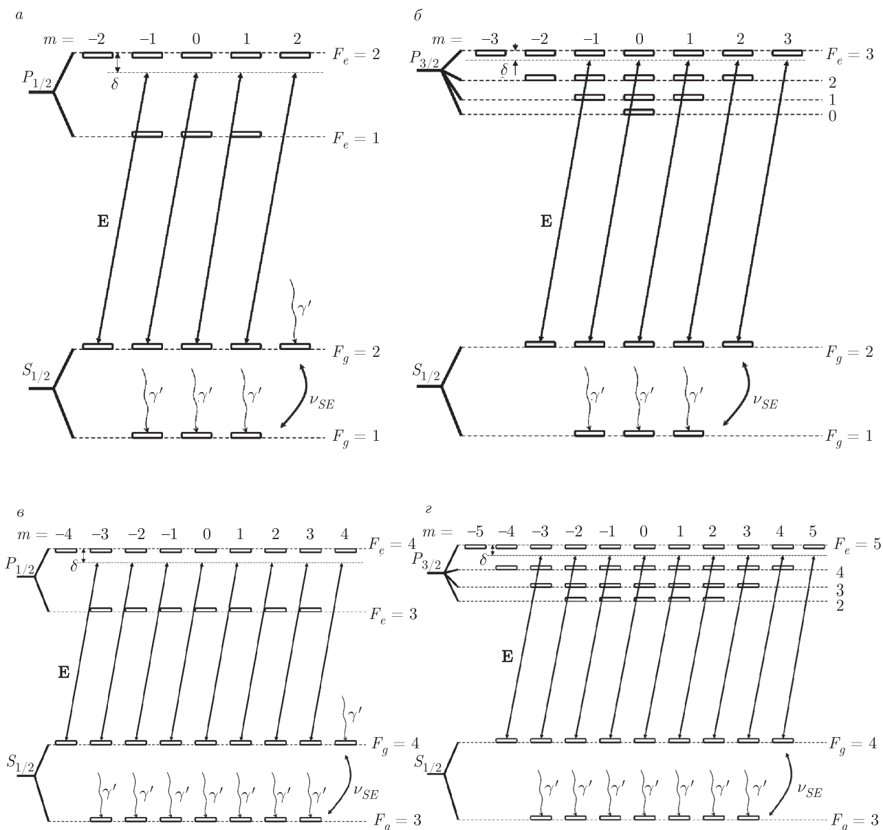
Рис. 1. Схемы возбуждения атома ^{87}\text{Rb} (а,б) и ^{133}\text{Cs} (в,г) на D_1 - и D_2 -линиях соответственно лазерным излучением \sigma^+ -поляризации, \delta — отстройка от перехода |F_g = I_n + J_g\rangle \leftrightarrow |F_e = I_n + J_e\rangle . \gamma' = (\gamma + \nu_Q)/N_g — результирующая скорость прихода из возбужденного состояния в основное
