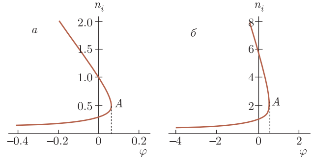
Рис. 6. Зависимости n_i(\varphi) (29) для адиабатических ИЗВ при \theta = 0.2 , \gamma_e = \gamma_i = 2 : a — случай периодических ИЗВ при V = 0.16 ; b — солитонный случай при V = 1.42
