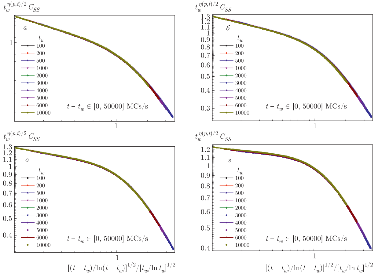
Рис. 11. Скейлинговые зависимости для автокорреляционной функции t_w^{\eta(p,T)/2} C_{SS}(t, t_w) в переменных [(t - t_w)/\ln(t - t_w)]^{1/2}/[t_w/\ln t_w]^{1/2} для чистой системы ( p = 1.0 ) с температурами замораживания T_s/T_{BKT} = 1.0 (а), 0.75 (б), 0.50 (в), 0.25 (г)
