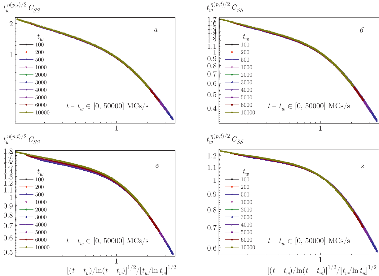
Рис. 12. Скейлинговые зависимости для автокорреляционной функции t_w^{\eta(p,T)/2} C_{SS}(t, t_w) в переменных [(t - t_w)/\ln(t - t_w)]^{1/2}/[t_w/\ln t_w]^{1/2} для структурно-неупорядоченной системы со спиновой концентрацией p = 0.9 и температурами замораживания T_s/T_{BKT} = 1.0 (а), 0.75 (б), 0.50 (в), 0.25 (г)
