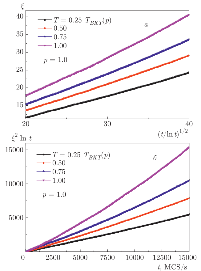
Рис. 3. Динамическая зависимость корреляционной длины \xi от (t/\ln t)^{1/2} (а) и величины \xi^2 \ln t от времени наблюдения t (б) при критической релаксации чистой двумерной XY -модели с линейным размером решетки L = 256 при t \leq 15000 MCS/s
