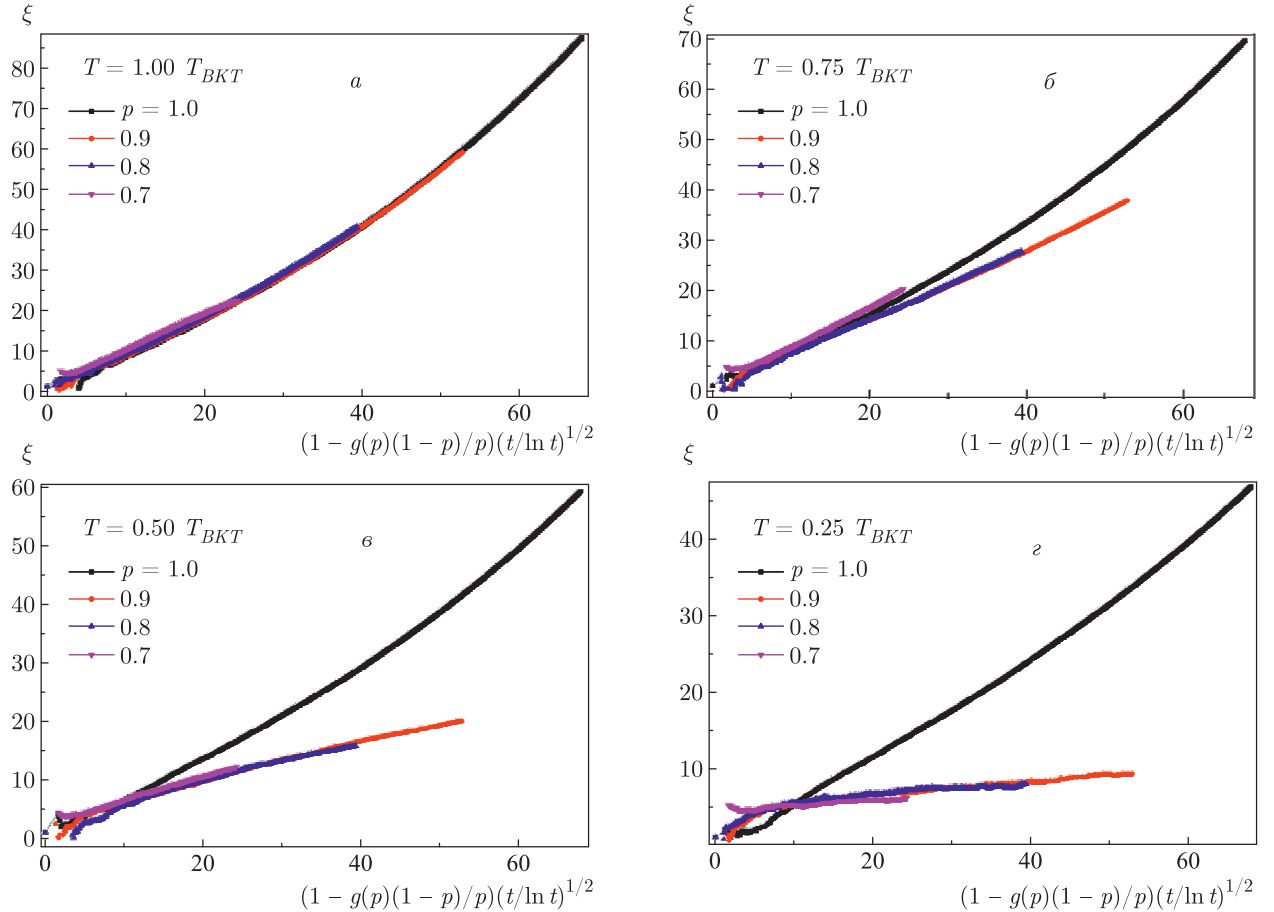
Рис. 4. Временная зависимость корреляционной длины \xi , построенная в переменных (1 - g(p)(1 - p)/p)(t/\ln t)^{1/2} , неравновесной критической релаксации чистой ( p = 1.0 ) и структурно-неупорядоченной ( p = 0.9, 0.8, 0.7 ) двумерной XY -модели на решетке с L = 256 ; температура замораживания системы T_s/T_{BKT} = 1.0 (а), 0.75 (б), 0.50 (в), 0.25 (г)
