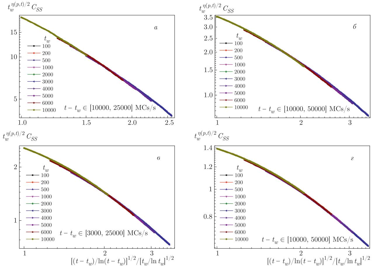
Рис. 14. Скейлинговые зависимости для автокорреляционной функции t_w^{\eta(p,T)/2} C_{SS}(t, t_w) в переменных [(t - t_w)/\ln(t - t_w)]^{1/2}/[t_w/\ln t_w]^{1/2} для структурно-неупорядоченной системы со спиновой концентрацией p = 0.7 и температурами замораживания T_s/T_{BKT} = 1.0 (а), 0.75 (б), 0.50 (в), 0.25 (г)
