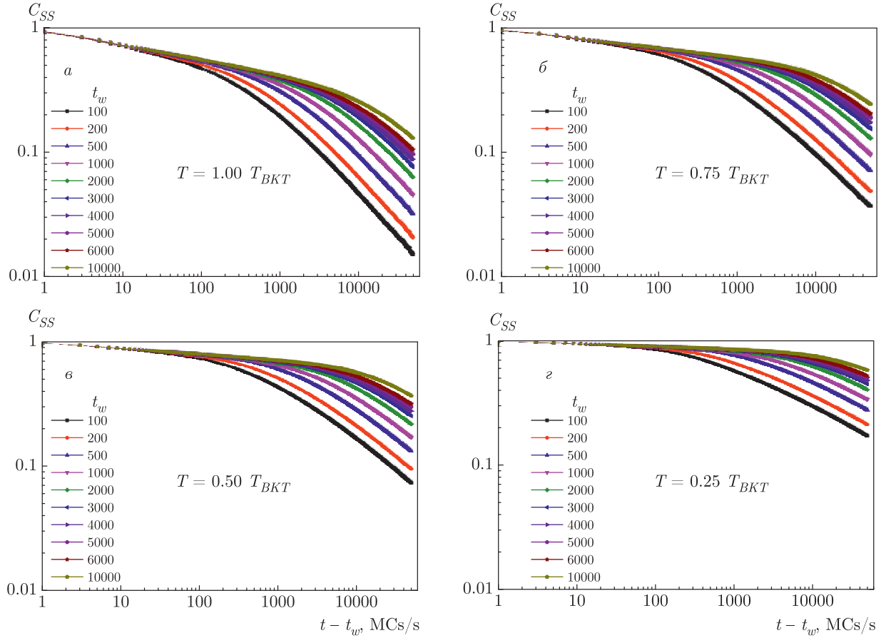
Рис. 8. Двухвременная зависимость спин-спиновой автокорреляционной функции C_{SS}(t, t_w) для структурно-неупорядоченной двумерной XY -модели со спиновой концентрацией p = 0.9 ; температуры замораживания T_s/T_{BKT} = 1.0 (а), 0.75 (б), 0.50 (в), 0.25 (г)
