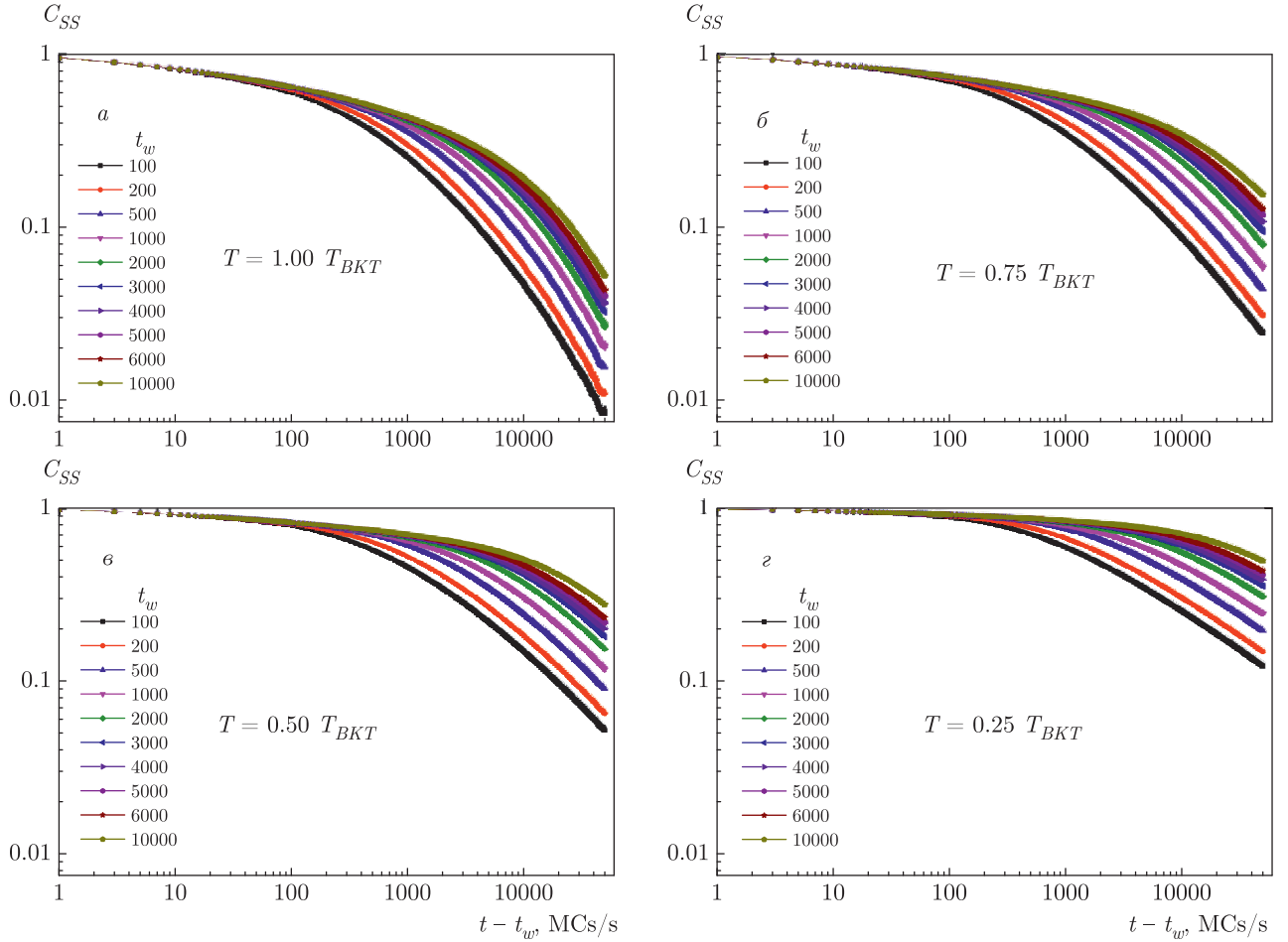
Рис. 10. Двухвременная зависимость спин-спиновой автокорреляционной функции C_{SS}(t, t_w) для структурно-неупорядоченной двумерной XY -модели со спиновой концентрацией p = 0.7 ; температуры замораживания T_s/T_{BKT} = 1.0 (а), 0.75 (б), 0.50 (в), 0.25 (г)
