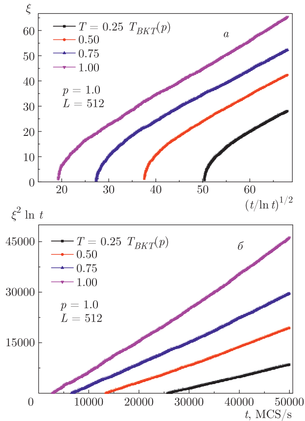
Рис. 2. Динамическая зависимость корреляционной длины \xi от (t/\ln t)^{1/2} (а) и величины \xi^2 \ln t от времени наблюдения t (б) при критической релаксации чистой ( p = 1.0 ) двумерной XY -модели с линейным размером решетки L = 512 ; время наблюдения t = 50000 MCS/s
