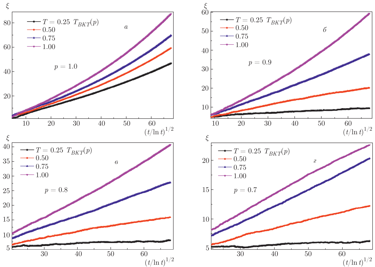
Рис. 1. Динамическая зависимость корреляционной длины \xi от (t/\ln t)^{1/2} при критической релаксации чистой ( p = 1.0 ) и структурно-неупорядоченной ( p = 0.9, 0.8, 0.7 ) двумерной XY -модели с линейным размером решетки L = 256 ; температура замораживания системы T_s/T_{BKT} = 1.0, 0.75, 0.50, 0.25 ; время наблюдения t = 50000 MCS/s
