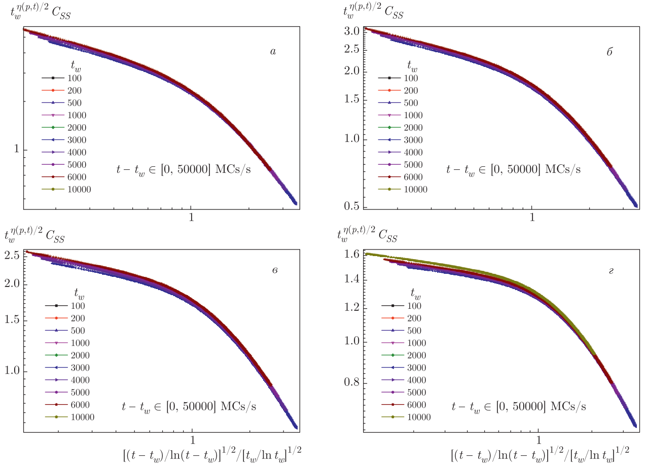
Рис. 13. Скейлинговые зависимости для автокорреляционной функции t_w^{\eta(p,T)/2} C_{SS}(t, t_w) в переменных [(t - t_w)/\ln(t - t_w)]^{1/2}/[t_w/\ln t_w]^{1/2} для структурно-неупорядоченной системы со спиновой концентрацией p = 0.8 , и температурами замораживания T_s/T_{BKT} = 1.0 (а), 0.75 (б), 0.50 (в), 0.25 (г)
