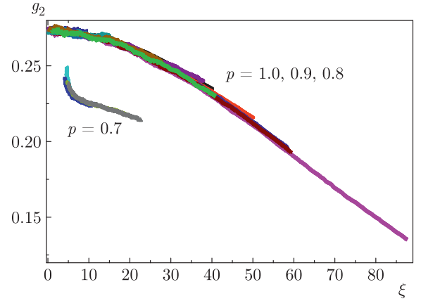
Рис. 6. Параметрическая зависимость кумулянта намагниченности g_2(t) от корреляционной длины \xi(t) для неравновесной критической релаксации двумерной XY -модели с концентрациями спинов p = 1.0, 0.9, 0.8, 0.7 при t \leq 50000 MCS/s; температуры замораживания системы T_s/T_{BKT} = 1.00, 0.75, 0.50, 0.25
