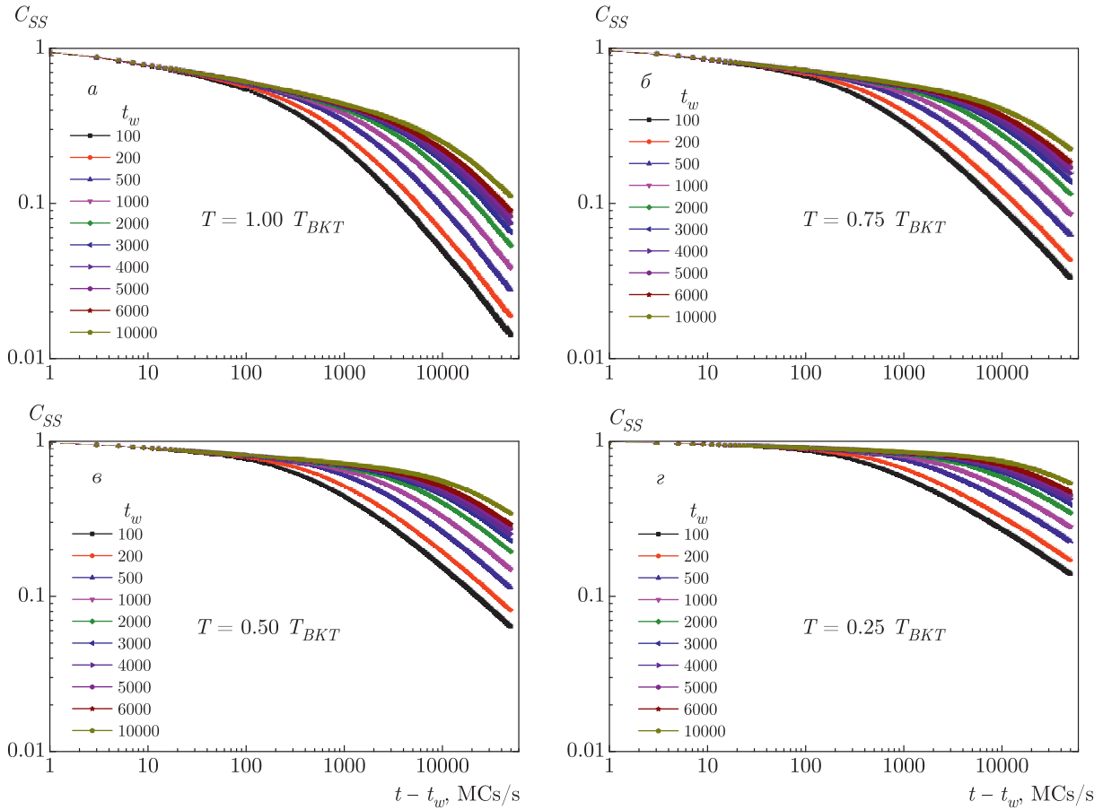
Рис. 9. Двухвременная зависимость спин-спиновой автокорреляционной функции C_{SS}(t, t_w) для структурно-неупорядоченной двумерной XY -модели со спиновой концентрацией p = 0.8 ; температуры замораживания T_s/T_{BKT} = 1.0 (а), 0.75 (б), 0.50 (в), 0.25 (г)
