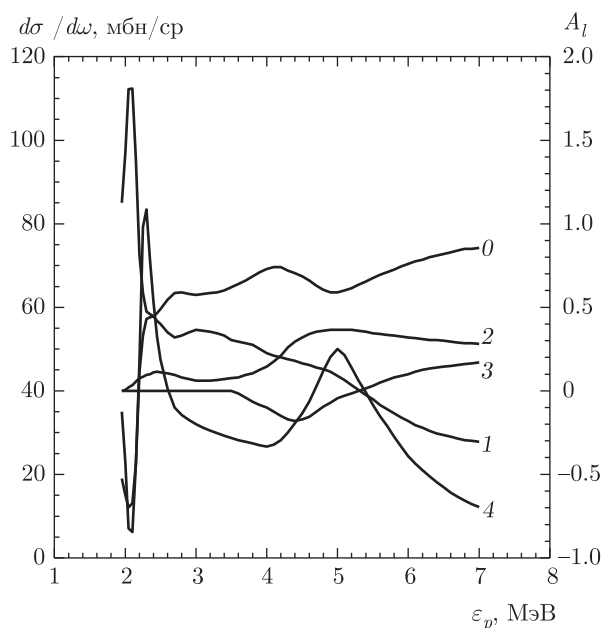
Рис. 4. Зависимости от энергии протона дифференциального сечения реакции {}^7\text{Li}(p, n){}^7\text{Be} при \mu = 1 (кривая 4) и коэффициентов A_l разложения этого сечения по полиномам Лежандра (кривые 0–3). Номера кривых A_l соответствуют номерам l полиномов P_l(\mu)
