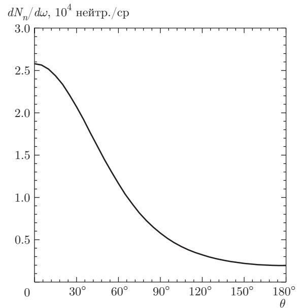
Рис. 7. Зависимость угловой плотности нейтронов от угла их вылета для моноэнергетичного пучка протонов с энергией \varepsilon_p = 2.4 МэВ, углом разброса направления их скоростей \theta_{ob} = 1^\circ и толщиной LiF-мишени 6.6 мкм
