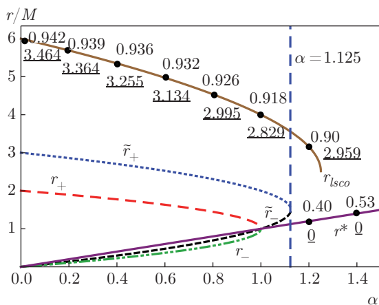
Рис. 15. Зависимости радиусов r_{lSCO}^+ , r_{lSCO}^- , \tilde{r}_+ , \tilde{r}_- , r_+ и r^* от параметра \alpha \in [0, 1.5] . Числа рядом с точками соответствуют значениям энергии E/\mu , а подчеркнутые числа — значениям момента импульса L/\mu M частицы для последней устойчивой круговой орбиты
