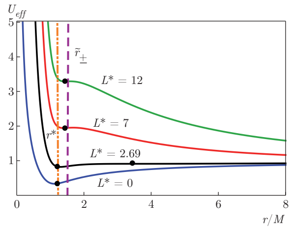
Рис. 10. Зависимости эффективного потенциала для случая III, \alpha = 9/8
