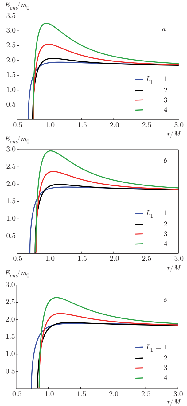
Рис. 18. Зависимости ЭЦМ при L_2 = 1 , 1 < \alpha G_N/G < 9/8 (а), \alpha G_N/G = 9/8 (б), \alpha G_N/G > 9/8 (е), случай III
